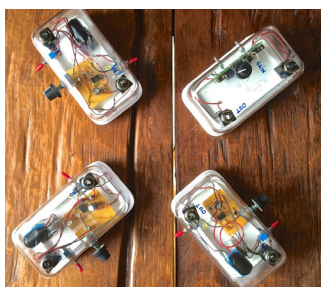
Lutherie électronique, 2016, installation sonore, quatre mini mapli fondés sur le lm386.
